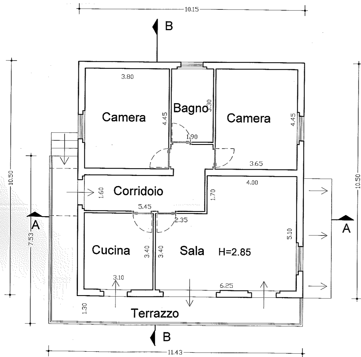
PIANTA TERRA
